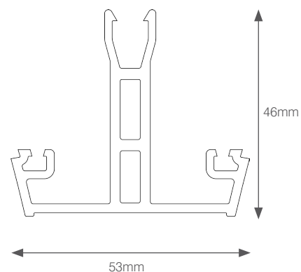
THERMAL T BAR KLP-09
