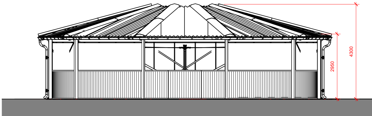
1 West 1 : 100
