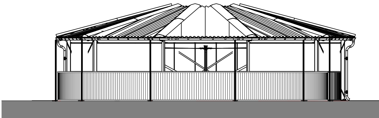
3 North 1 : 100
