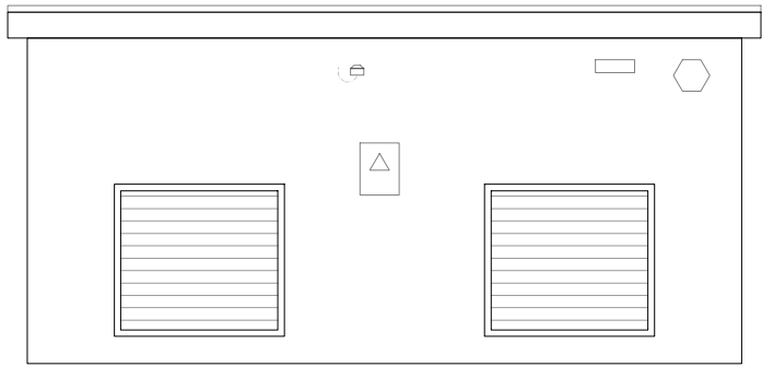
Elevation 4
