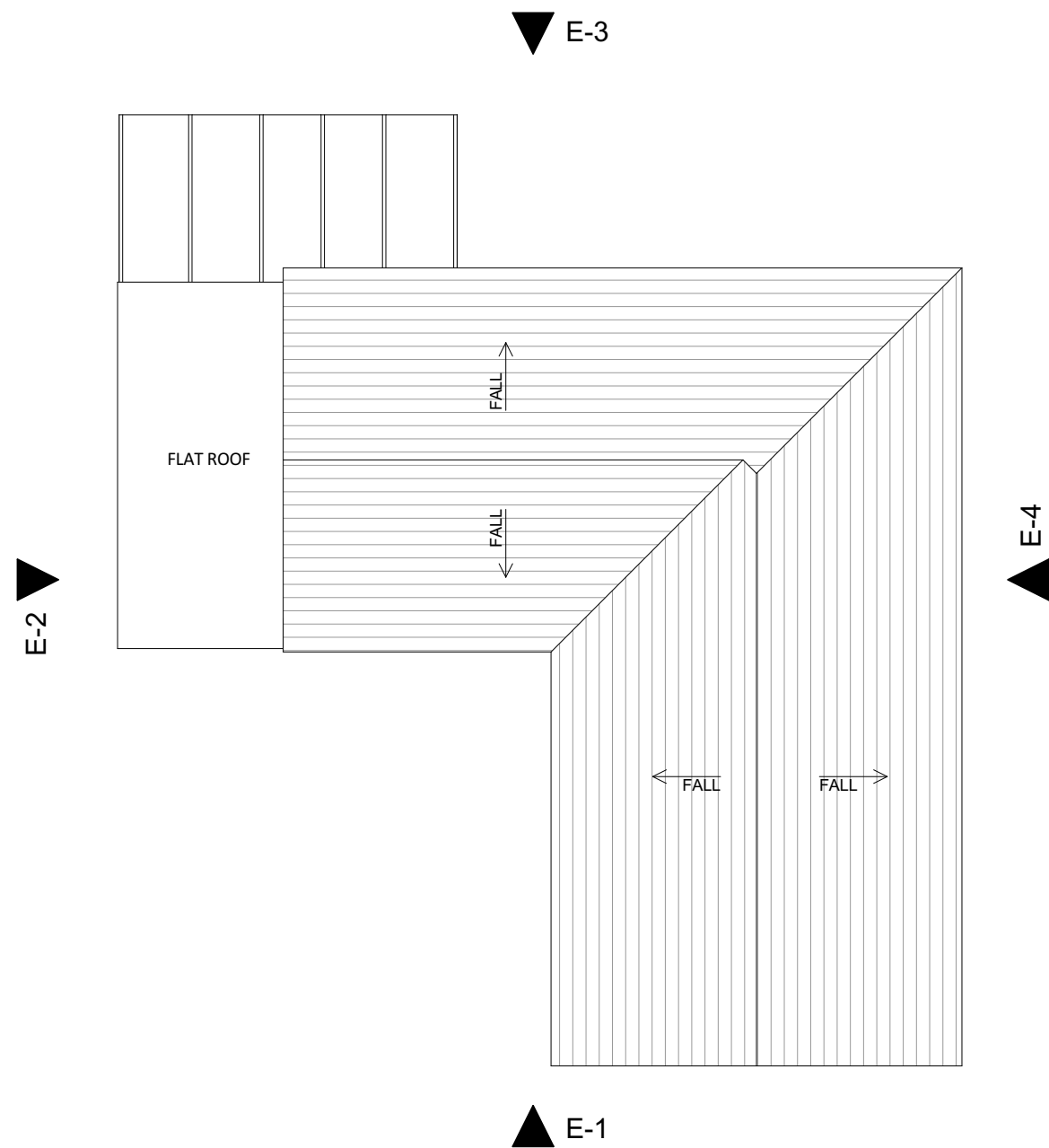
2 RF-Roof 1:100
