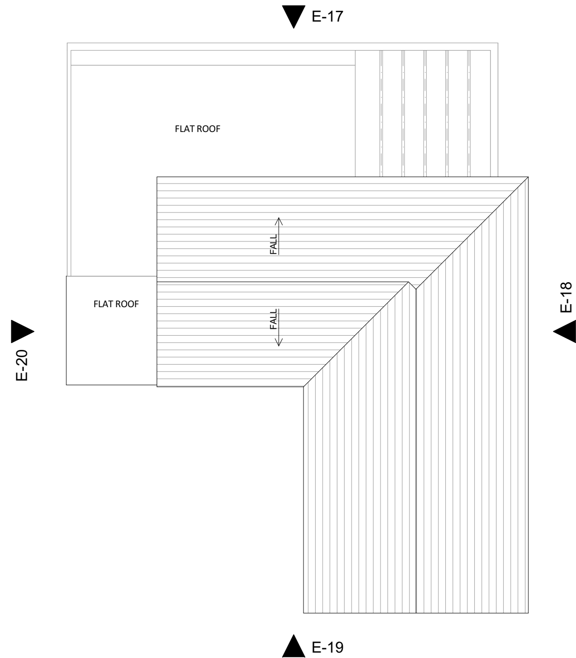
2 RF-Roof 1:100
