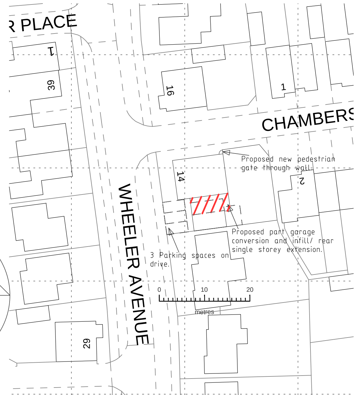
Site Plan 1 : 500
