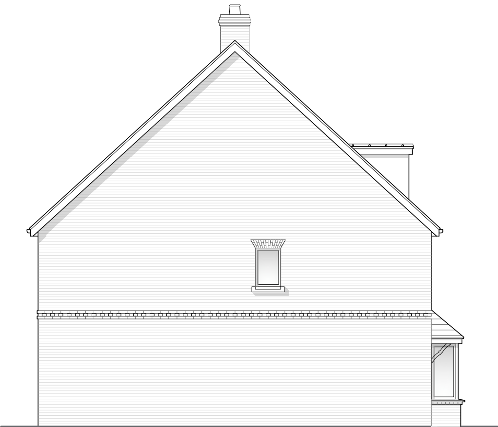
Elevation B
