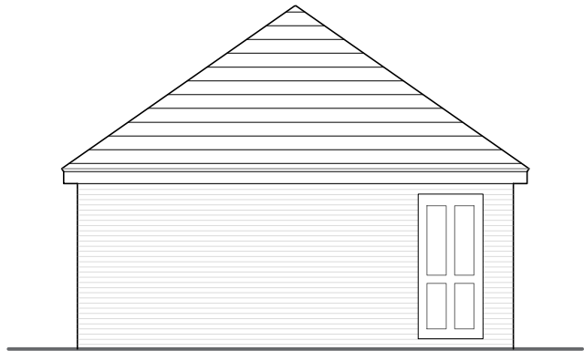
Elevation B
