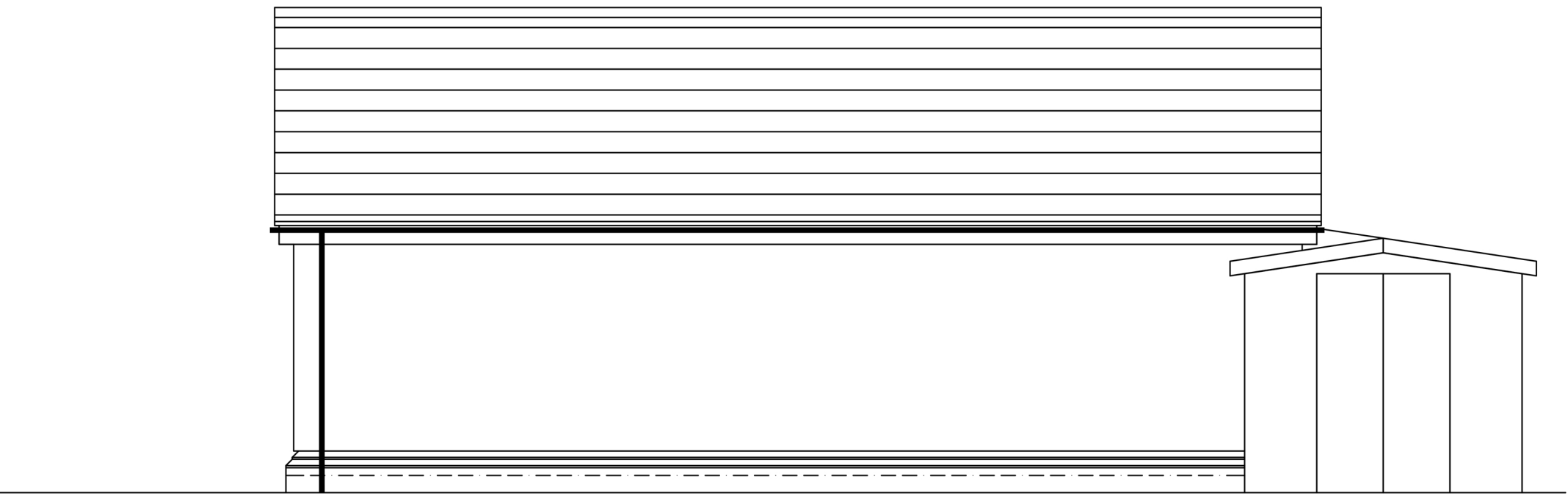
ELEVATION `C`
