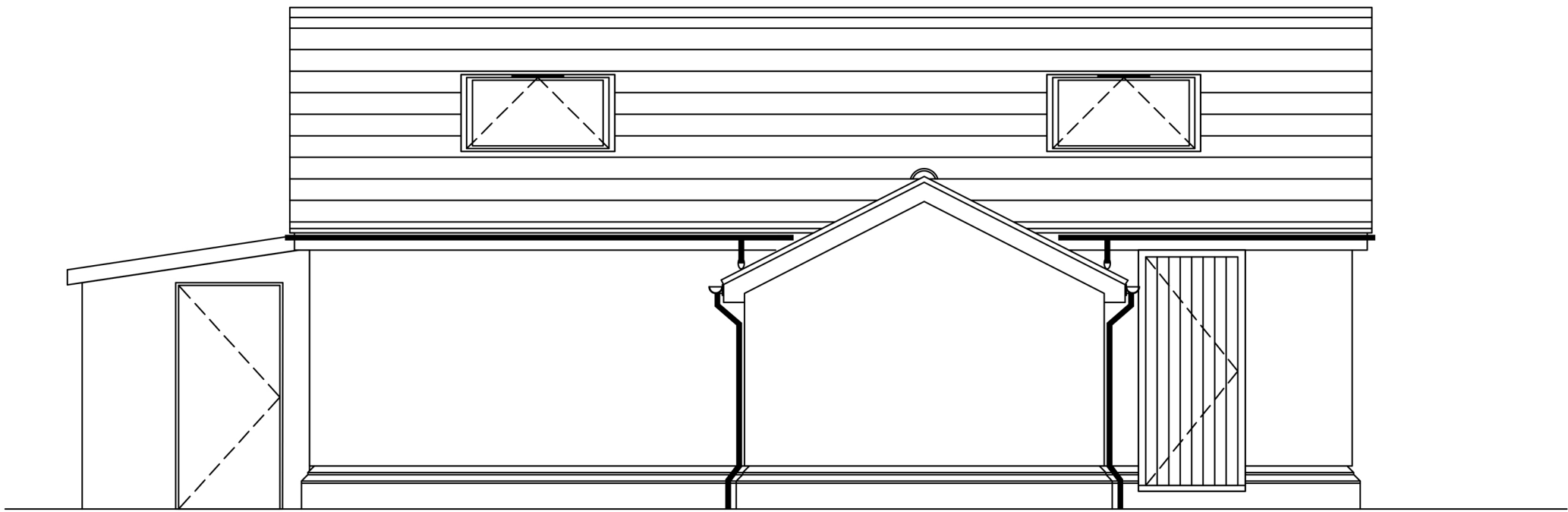
ELEVATION `A`
