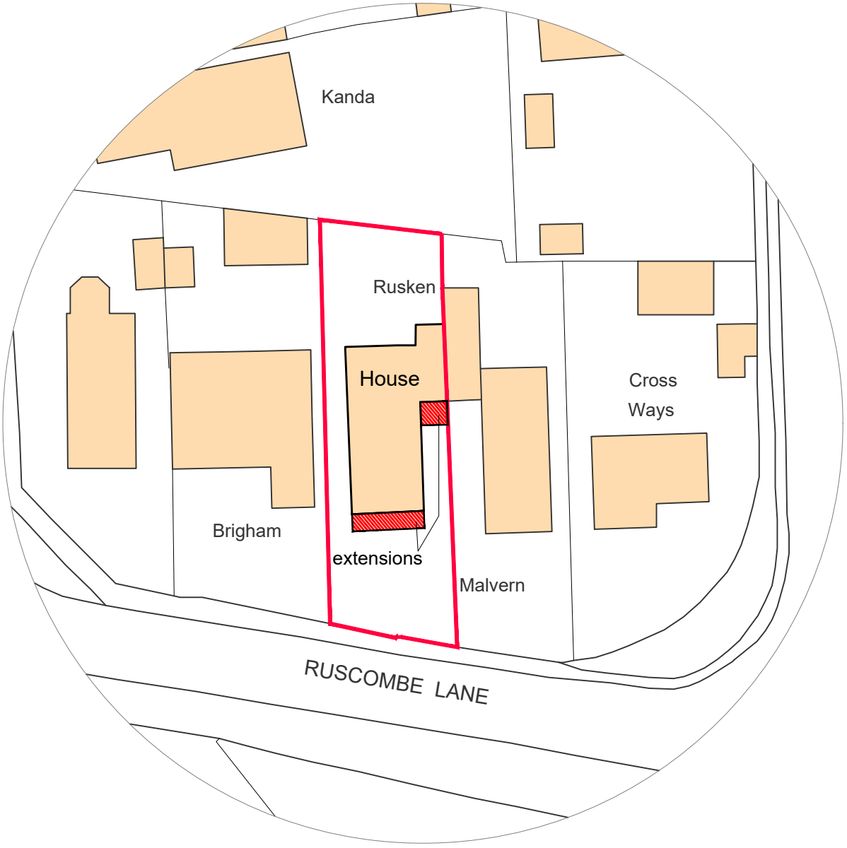
Block Plan 1 : 500
