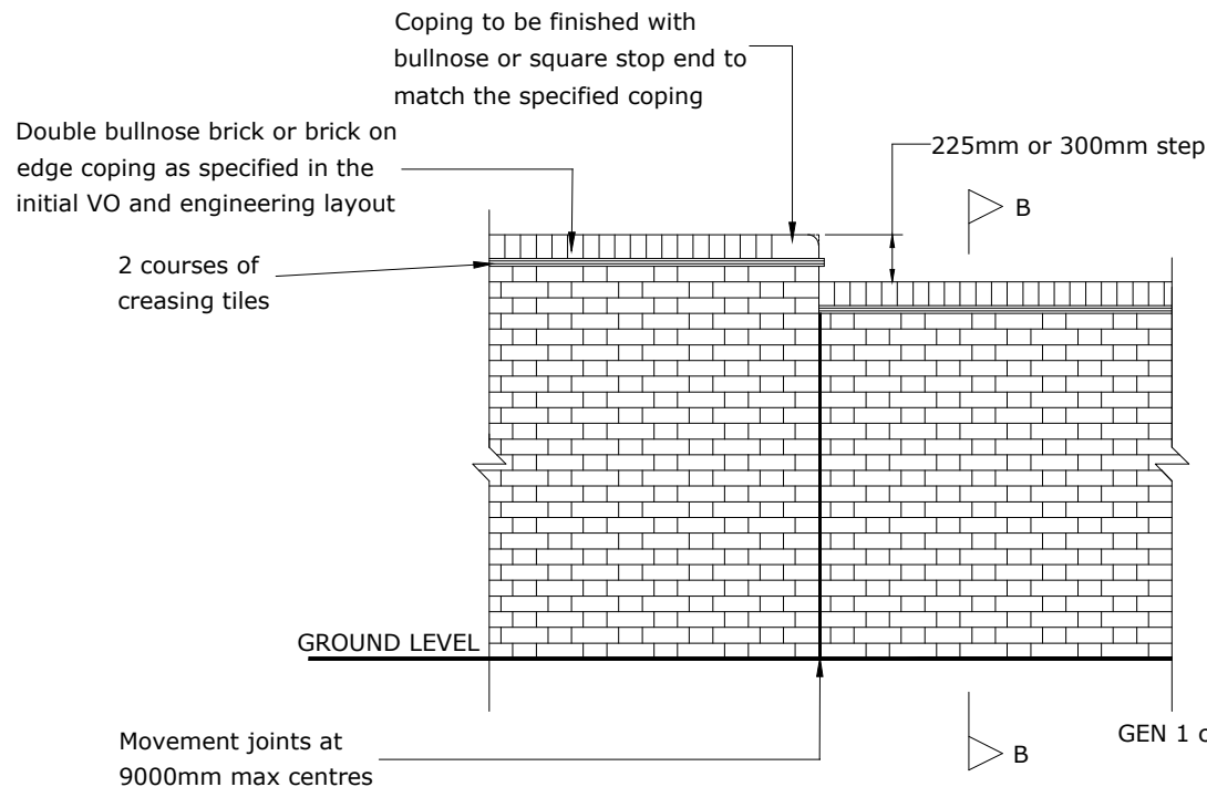
ELEVATION
